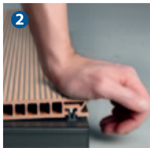
2 Anfangsclip auf der Unterkonstruktion festschrauben und erste Bodendiele einrasten.
