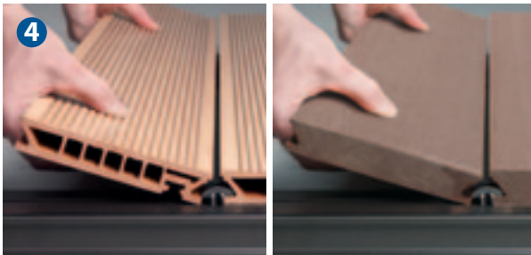
Folgende Bodendielen einschieben.
