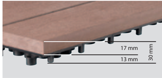
geringe Aufbauhöhe
