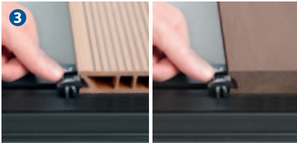
Zur weiteren Montage der Dielen Montageclips einfügen – ohne zu schrauben!
