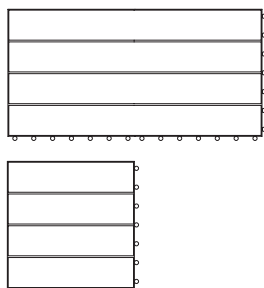
linke Fliese 364 x 728 / 364 x 364
